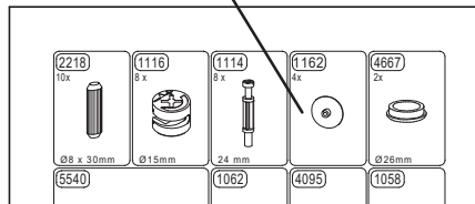
Beschlagteile/ fittings
